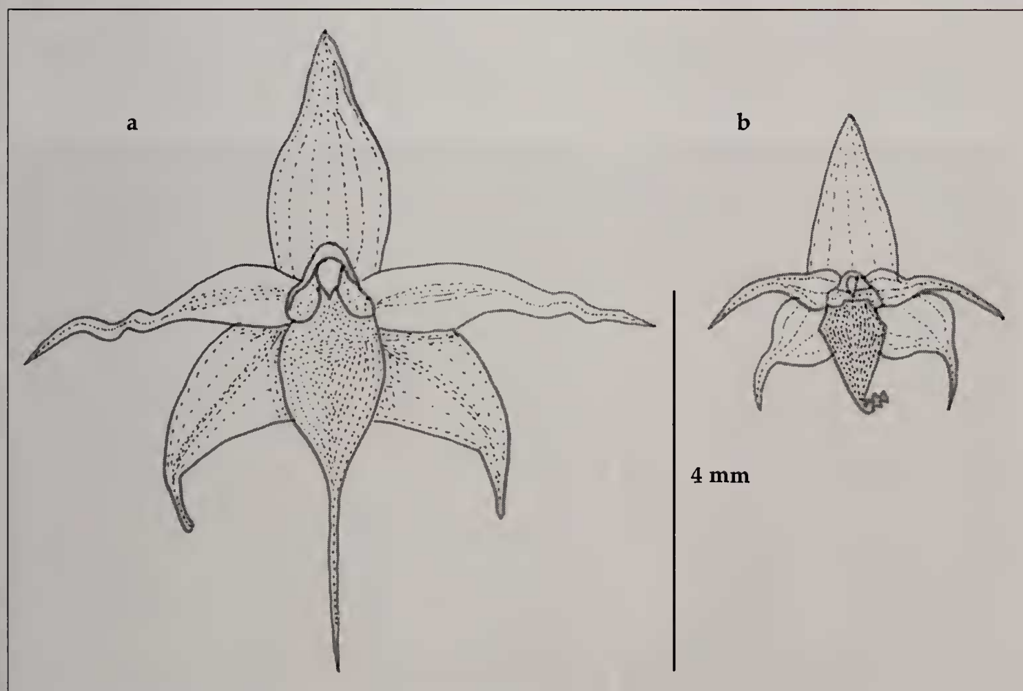
Fig. 2 : Platystele ovipositoglossa [a] & Platystele crotaloglossa [b] dessin F.Archila
